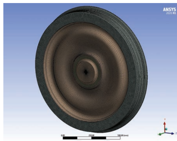
Rys. 4. Model 3D koła – siatka [opracowanie własne]
