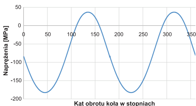
Rys. 15. Historia na naprężeń z przykładowej współosiowej grupy punktów [opracowanie własne]
