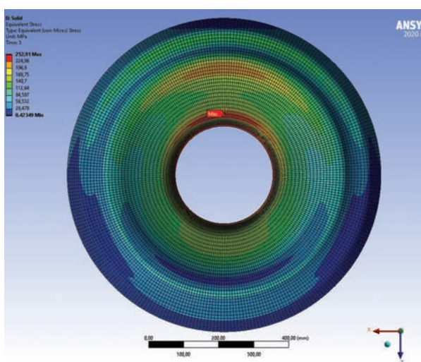
Rys. 9. Model 3D: przypadek obciążenia 2 – naprężenia Hubera [opracowanie własne]
