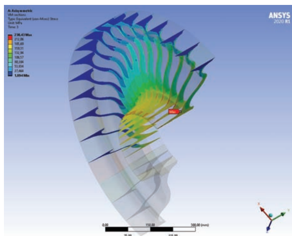
Rys. 13. Model osiowosymetryczny: przypadek obciążenia 2 – naprężenia Hubera [opracowanie własne]
